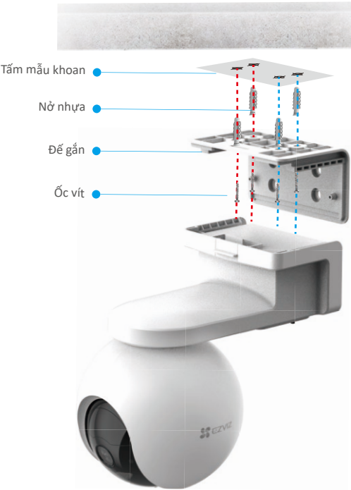
Hình 1 Gắn trần
