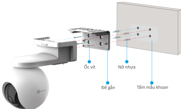
Hình 2 Gắn tường
